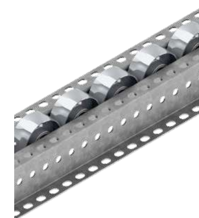
▶ Rueda INTERFLO de Aluminio para Alto Impacto \varnothing 2.875''
