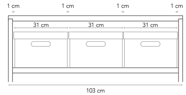
Entrepaños para cajas tamaño carta
